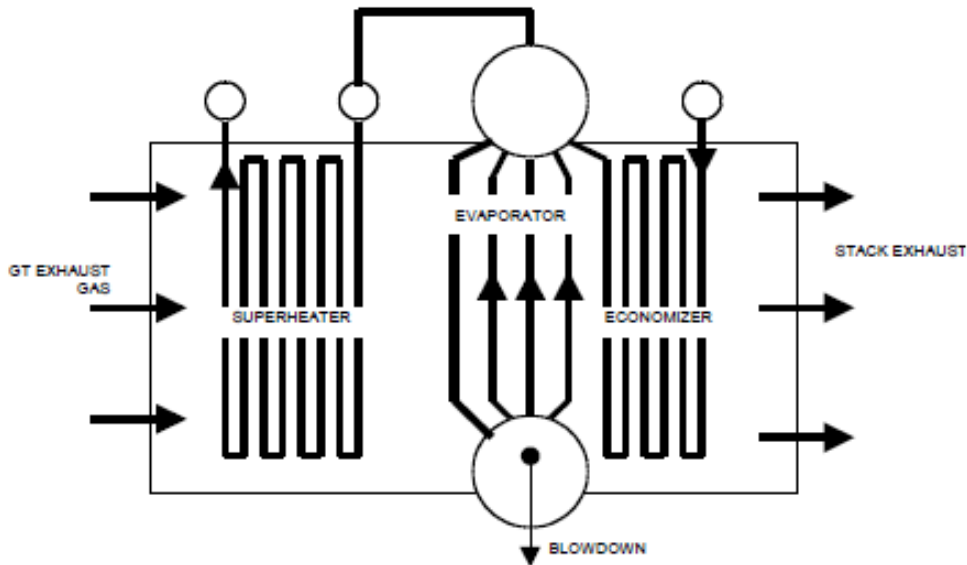
Figure 2: Drum-Type HRSG
